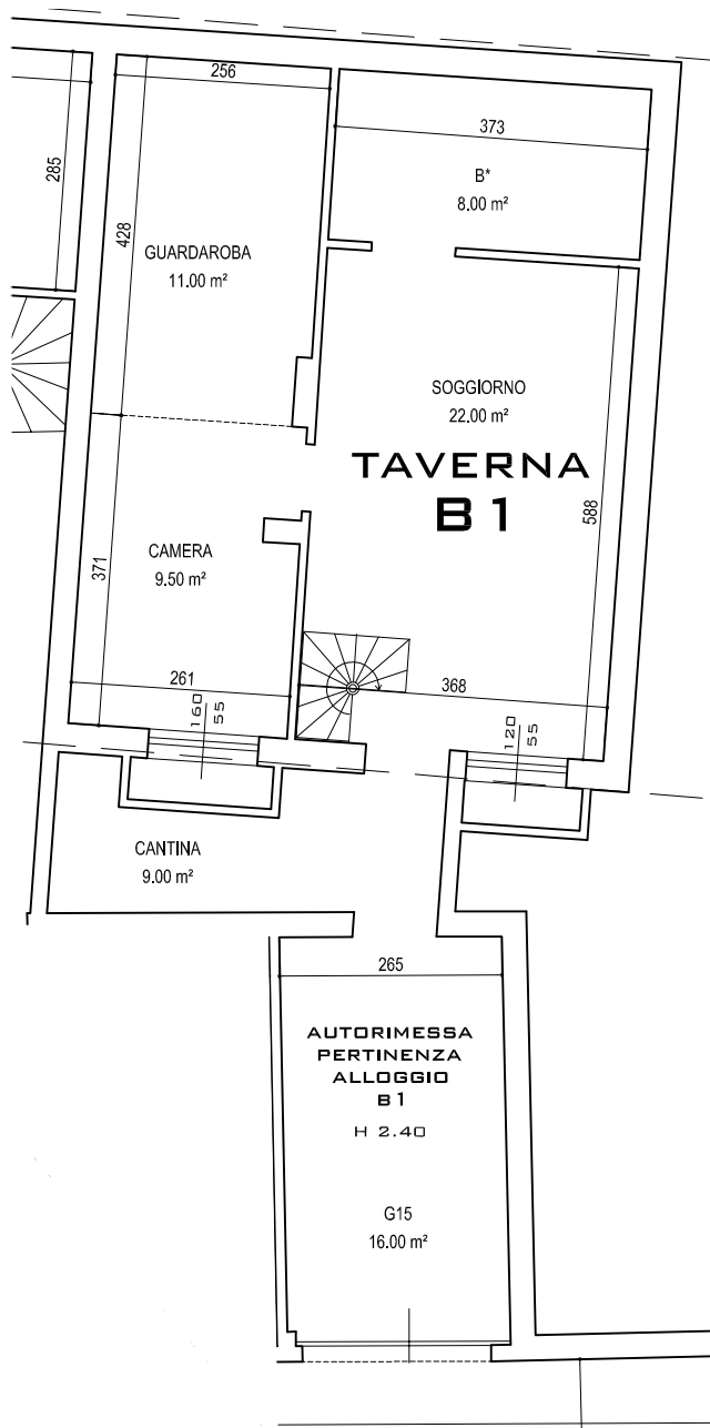
TAVERNA E AUTORIMESSA PIANTA PIANO INTERRATO
